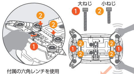
付属の六角レンチを使用
